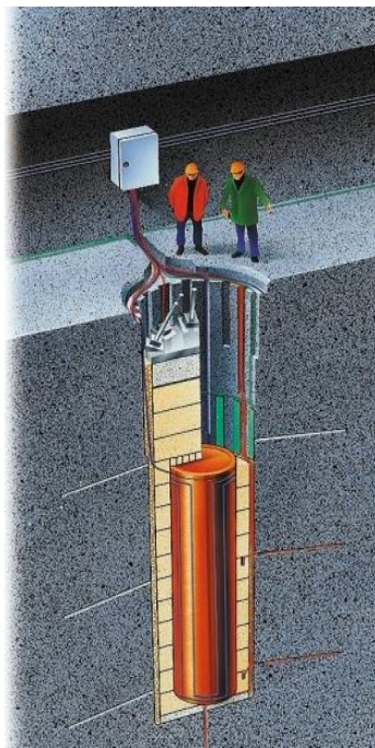
Essai de dépose des anneaux de bentonite en vue de la récupération de colis de déchets* en Suède (Äspö HRL, 2006)
